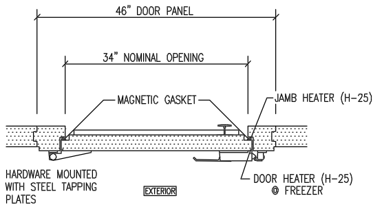
SECTION DOOR PANEL
