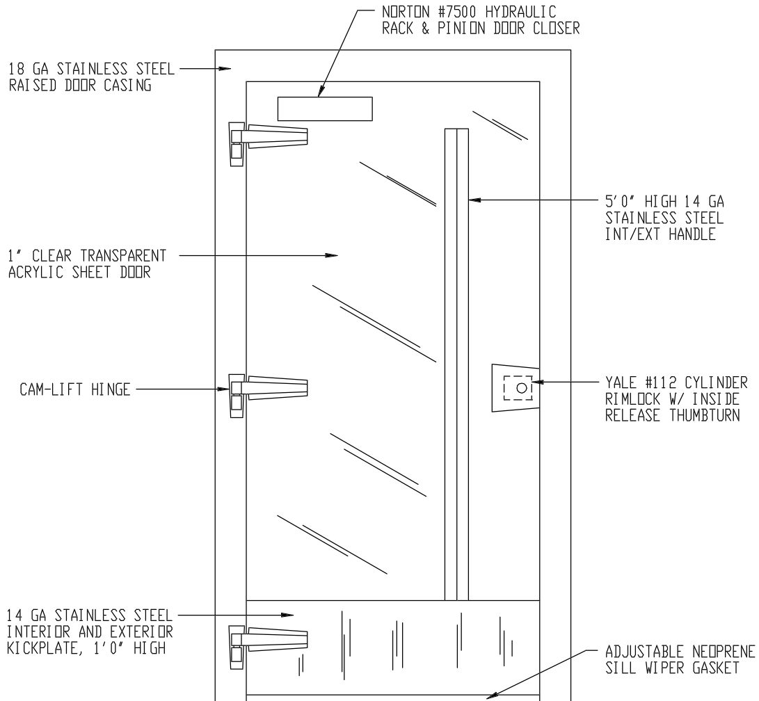
DOOR ELEVATION
